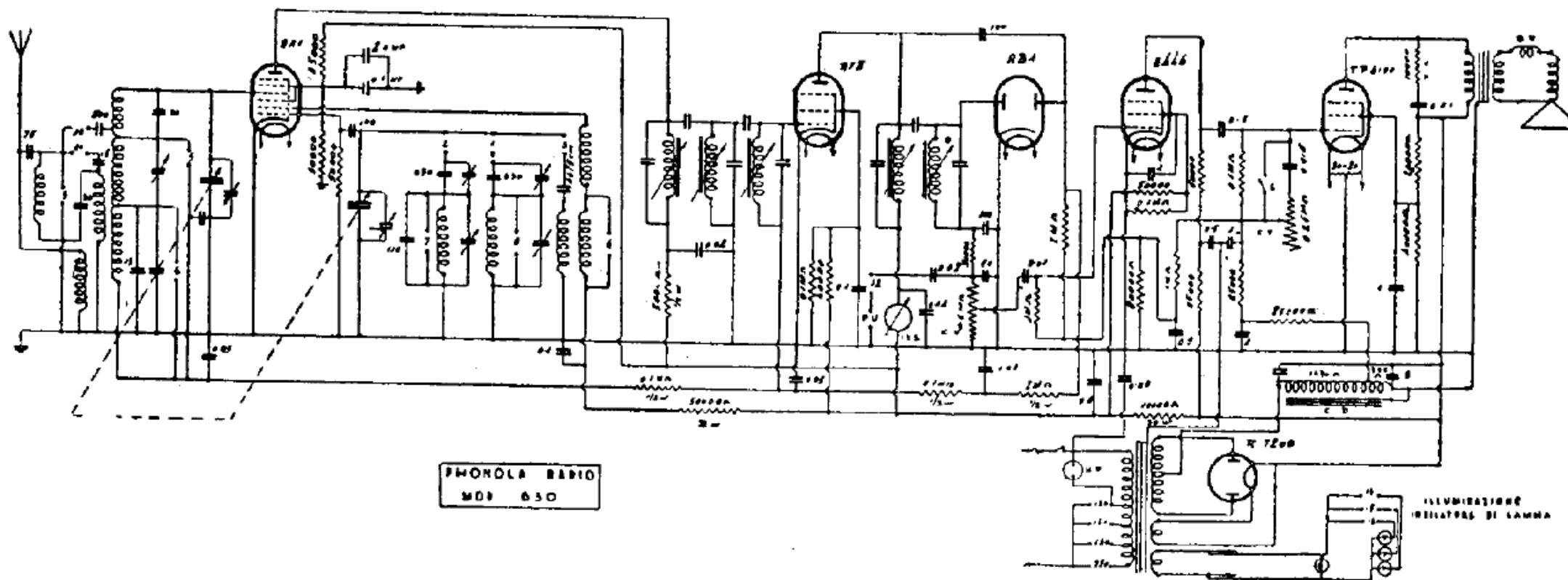
PHONOLA-RADIO (S A FIMI) — Modelli « 630, 631, 632 e 633 » - Produzione 1934. - Media frequenza: 175 kc.
